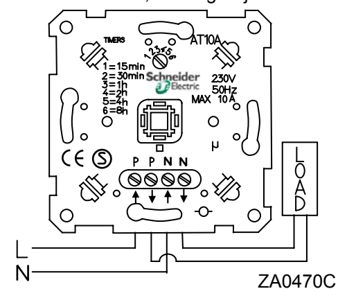
Wiring diagram, Kopplingschema Johdotuskaavio, Koblingskjema
